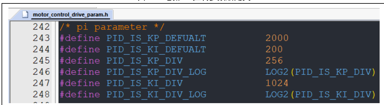
图 24. 电流 PI 控制参数宏定义
