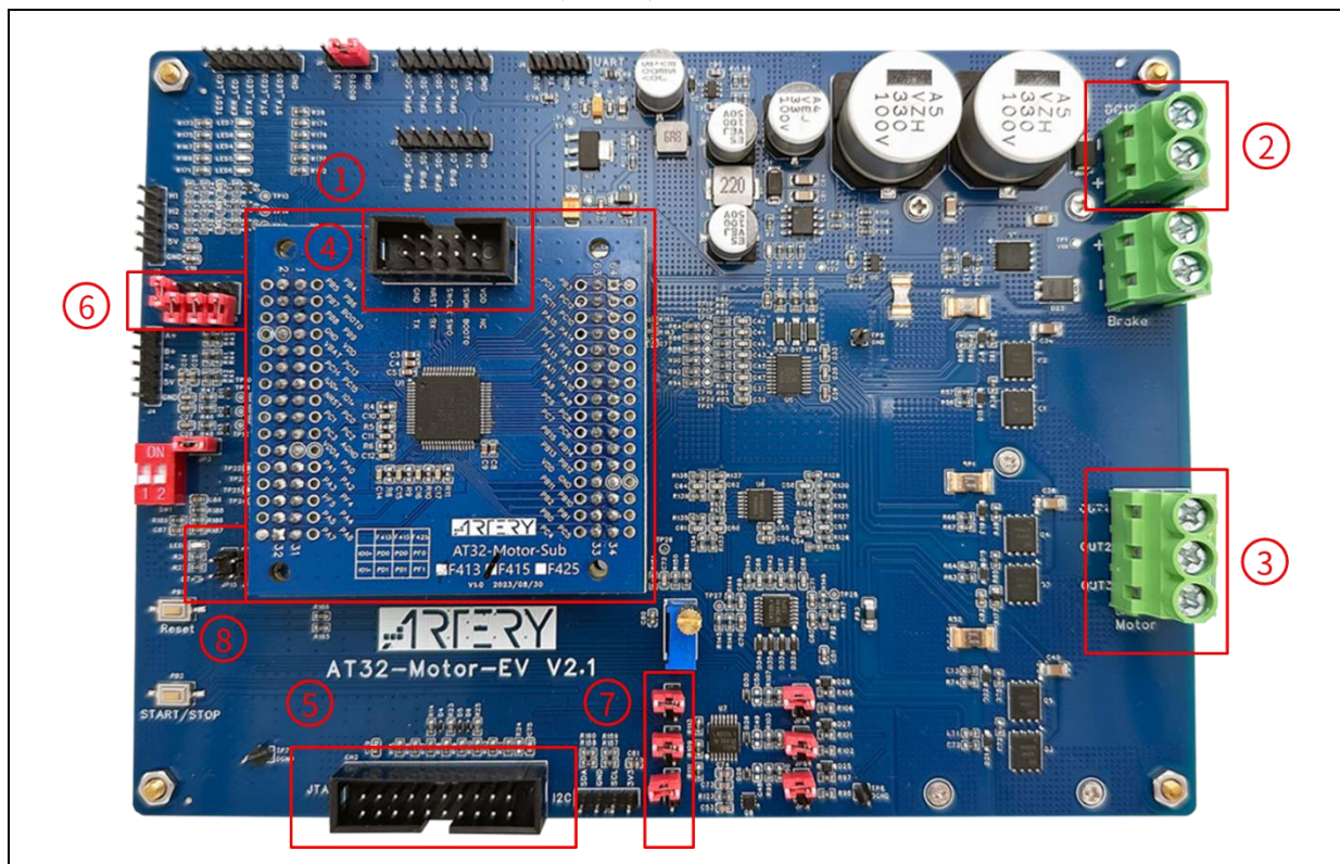
图 1. 电机开发板 AT-MOTOR-EVB
