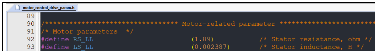
图 15. 电机线圈参数宏定义
