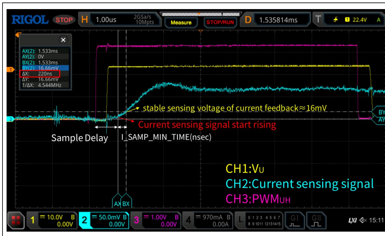
图 11. 电流取样延迟时间测量波形
