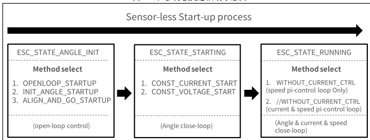
图 27. 六步方波无感启动示意图
