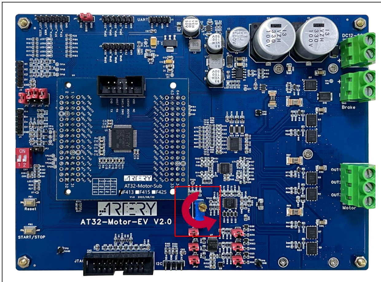
图 42. 电位器位置图（外部电压控制来源）
