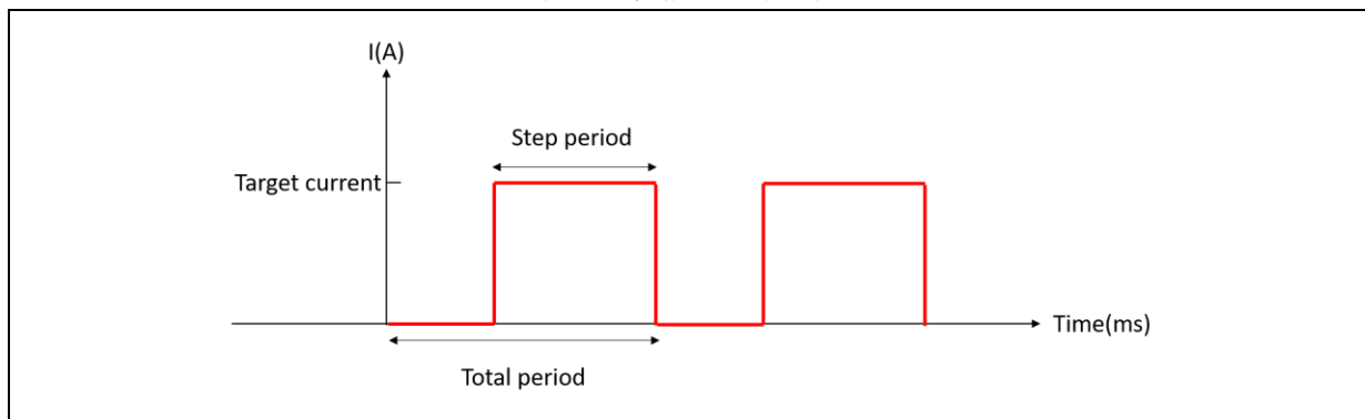
图 19. 步阶电流示意图
