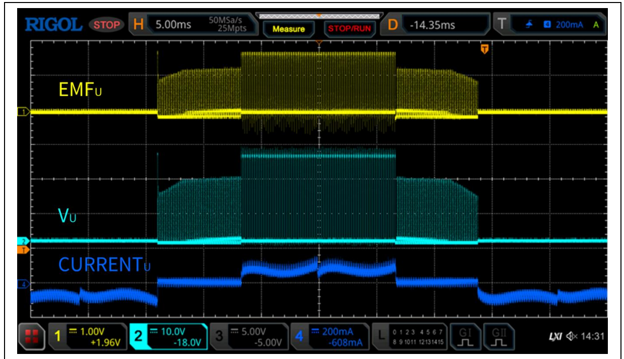
图 31. 反电势对称波型图
