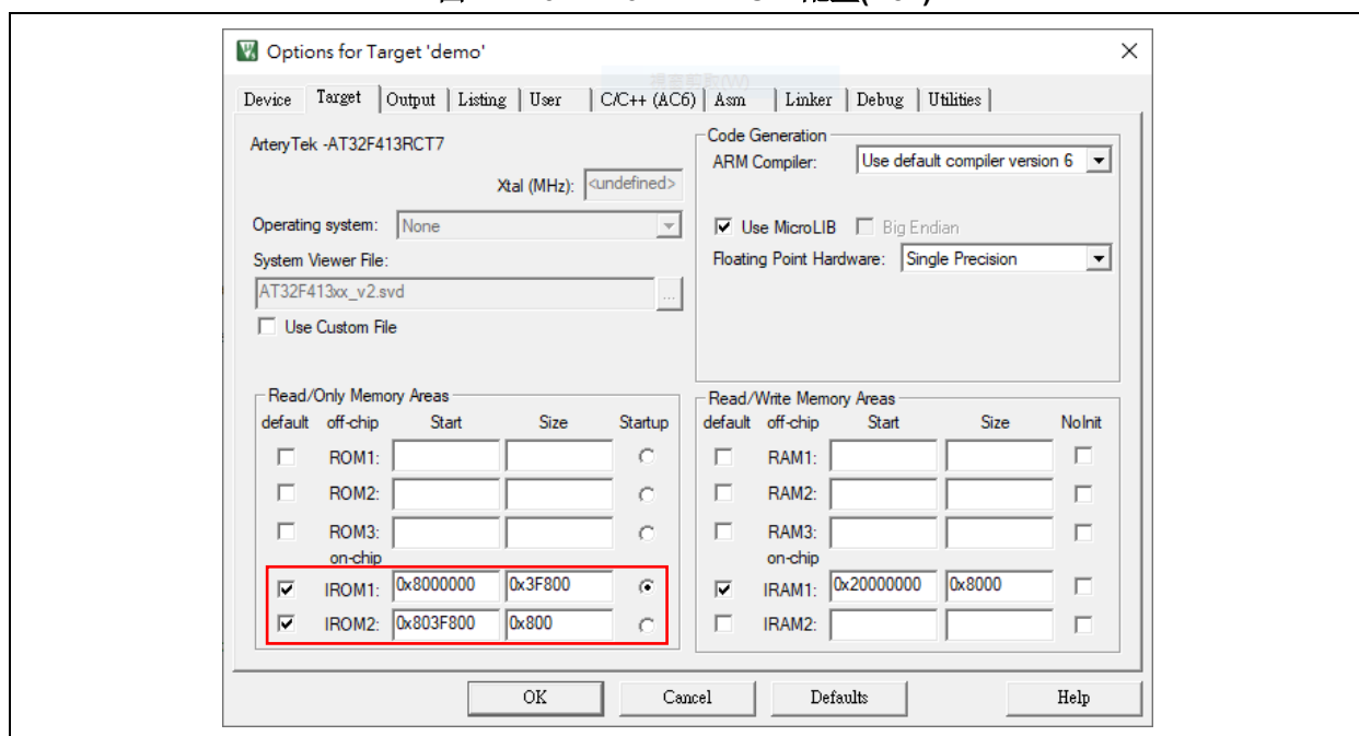
图 2. AT32F413RCT7 ROM 配置(Keil)
