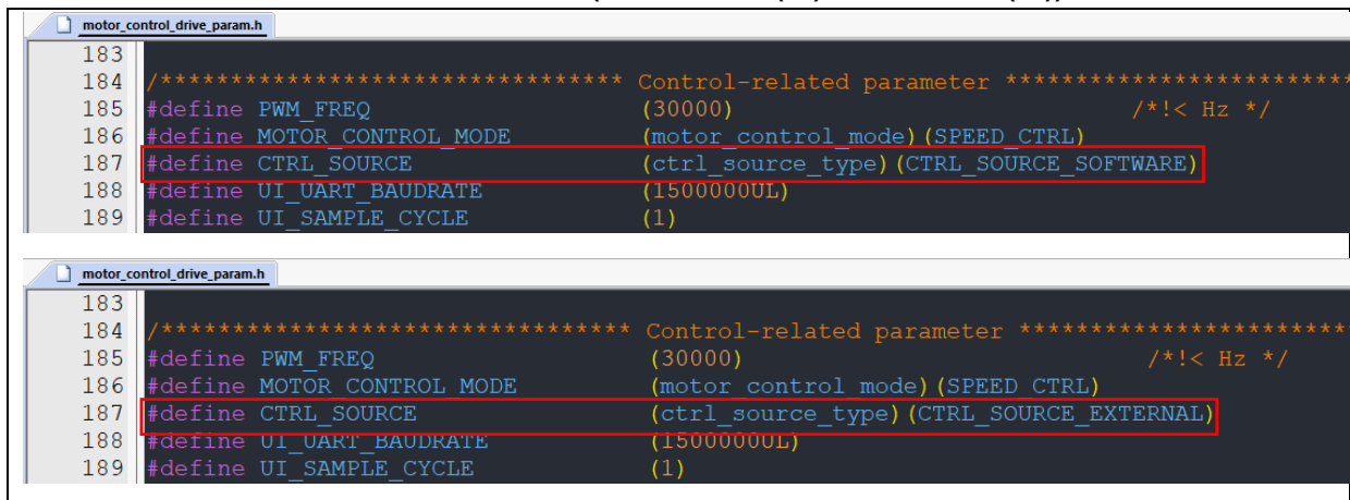
图 43. 控制来源定义值(软件控制来源(上)/外部电压控制(下))
