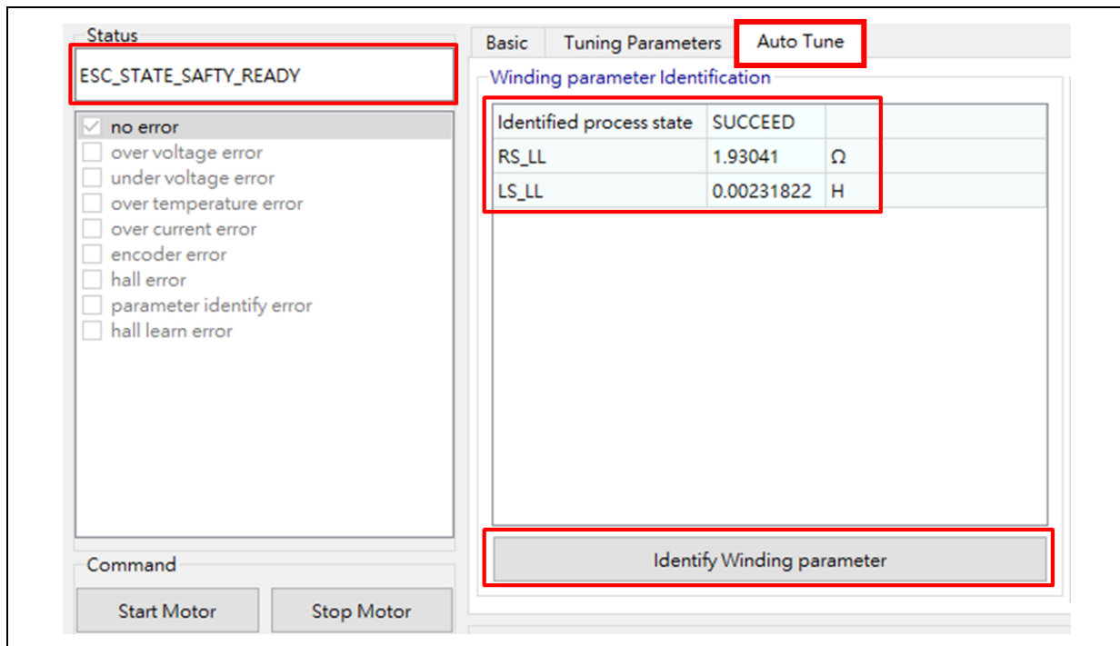
图 14. 电机线圈参数自动辨识
