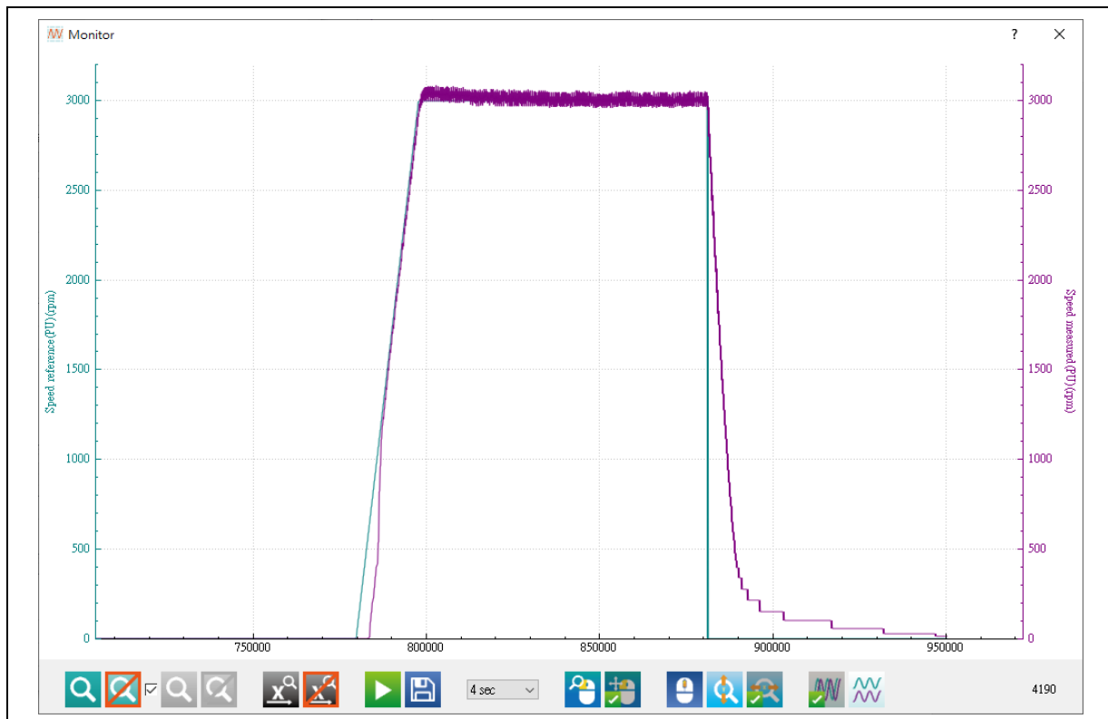
图 35. 速度环调试波形
