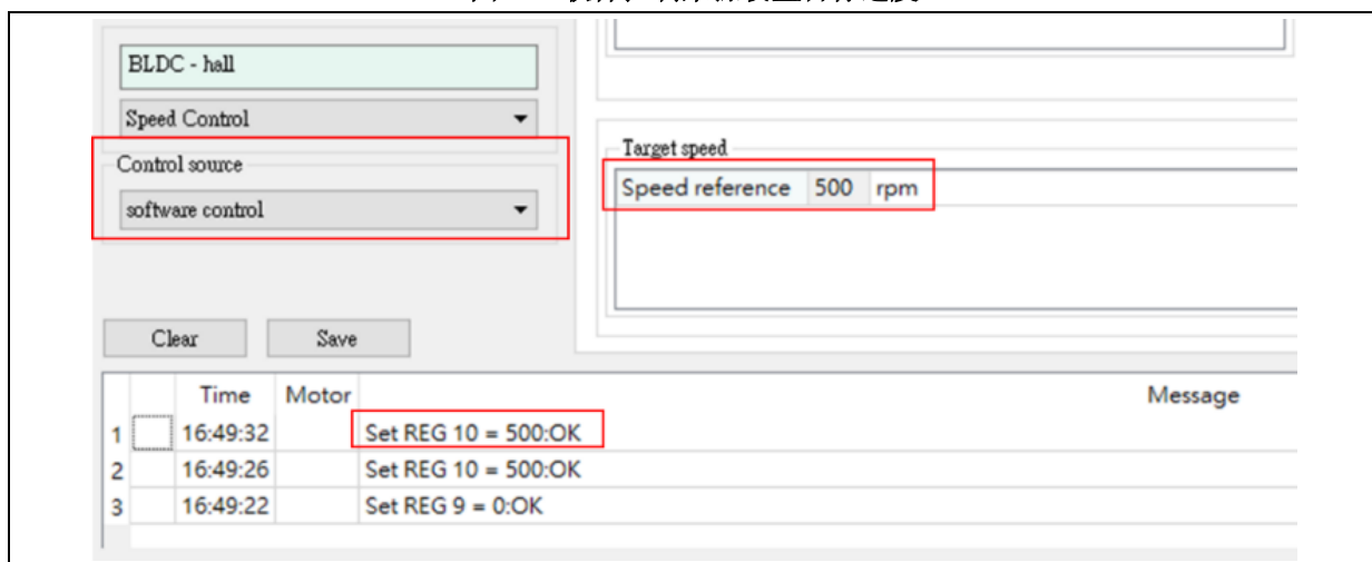
图 46. 软件控制来源设置目标速度
