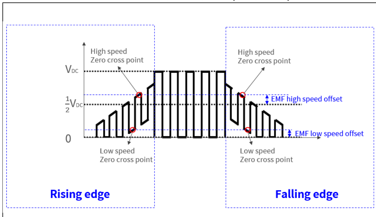
图 30. 六步方波反电势调试参数示意图(ADC 检测方法)
