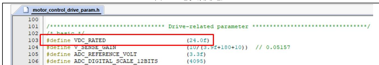
图 16. 电机额定电压
