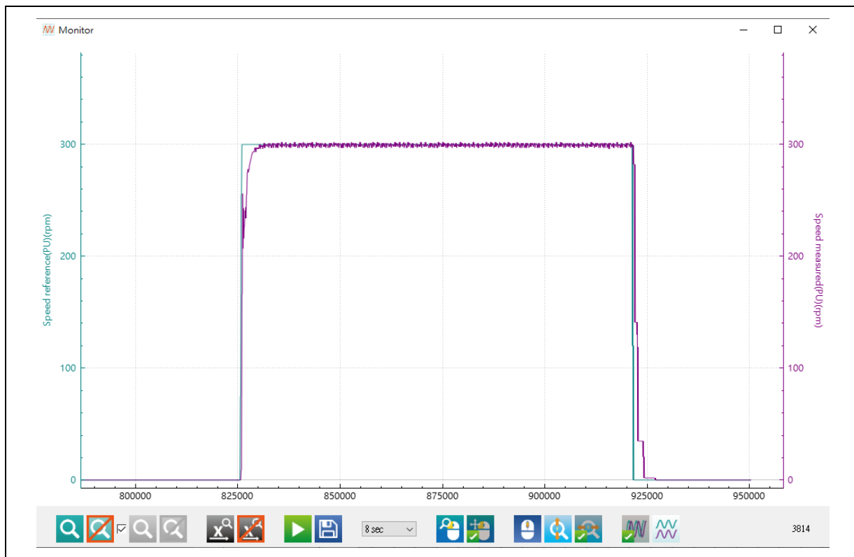
图 41. 速度电压环调试波形
