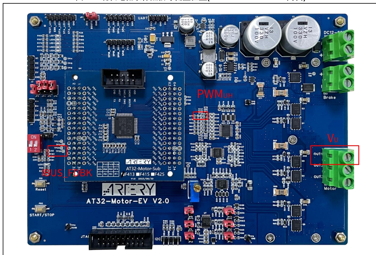
图 10. 确认电流取样点信号测量位置(AT32-Motor-EVB2.0 为例)
